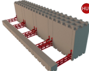
IsoteQ ® EXTRA Koszorúelem
